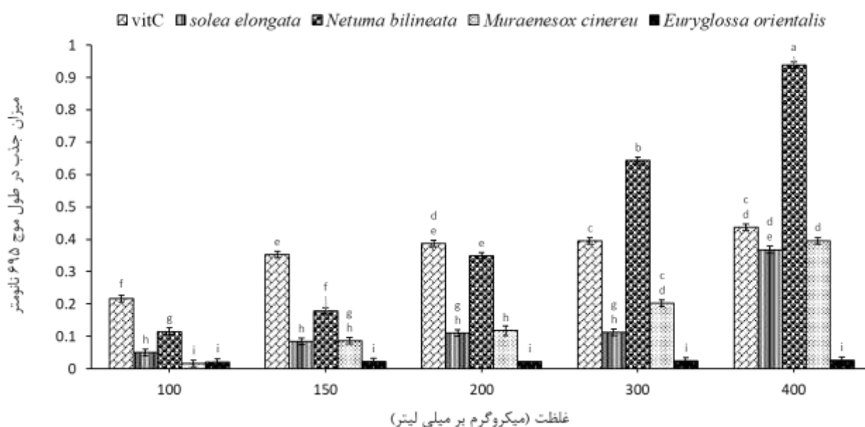
شکل ۲. مقایسه ظرفیت ضداکسیدانی مخاط چهار گونه ماهیان مورد مطالعه در غلظت‌هایی مختلف با آسکوربیک اسید به عنوان استاندارد. حروف غیرمشابه بیانگر وجود اختلاف معنی‌دار بین نمونه‌ها است ( P \leq 0/05 ).
