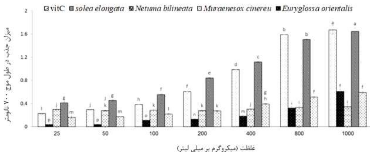
شکل ۱. مقایسه توان احیاکنندگی مخاط چهار گونه ماهیان مورد مطالعه در غلظت‌های مختلف با آسکوربیک اسید به عنوان استاندارد. حروف غیرمشابه بیانگر وجود اختلاف معنی‌دار بین نمونه‌ها است ( P \leq 0/05 ).
