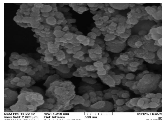
\gamma\text{-Fe}_2\text{O}_3\text{@SiO}_2\text{@TiO}_2\text{-Ni}
