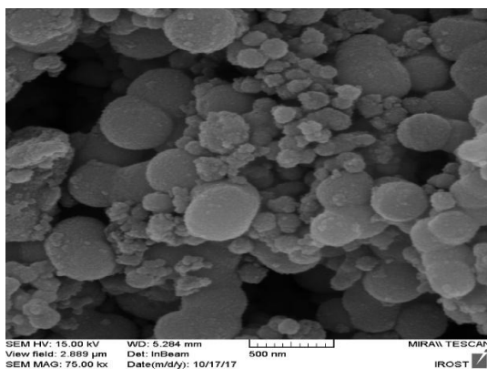
\gamma\text{-Fe}_2\text{O}_3@SiO_2@TiO_2\text{-Cu}
