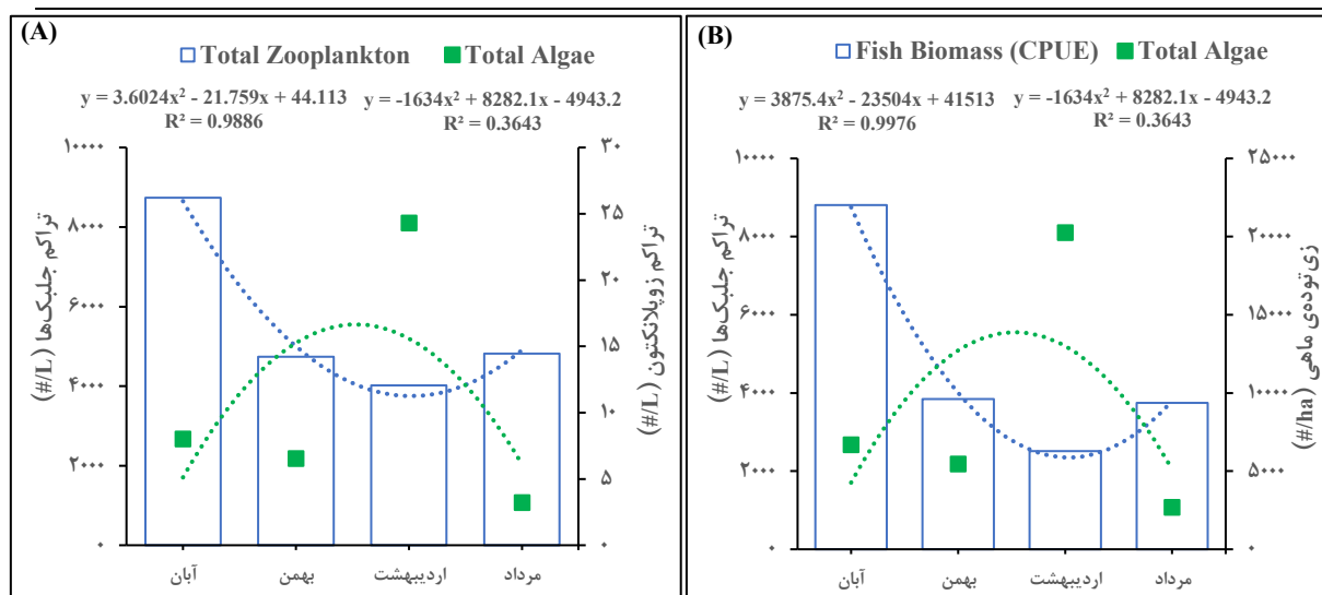
شکل ۵: روند تغییر سالانه‌ی جمعیت فیتوپلانکتون‌ها با عامل‌های زیستی: زئوپلانکتون (A) و ماهی (B).
