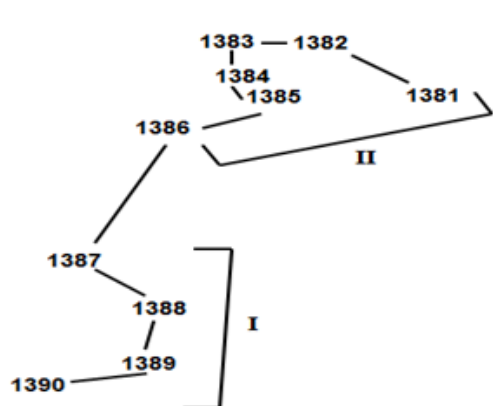
شکل ۵. دندوگرام آنالیز خوشه‌ای و دسته‌بندی غیرمتریک (nMDS) ترکیب صید آبهای استان هرمزگان (۹۰-۱۳۸۱) و تفکیک آن به دو گروه سالی I و II
