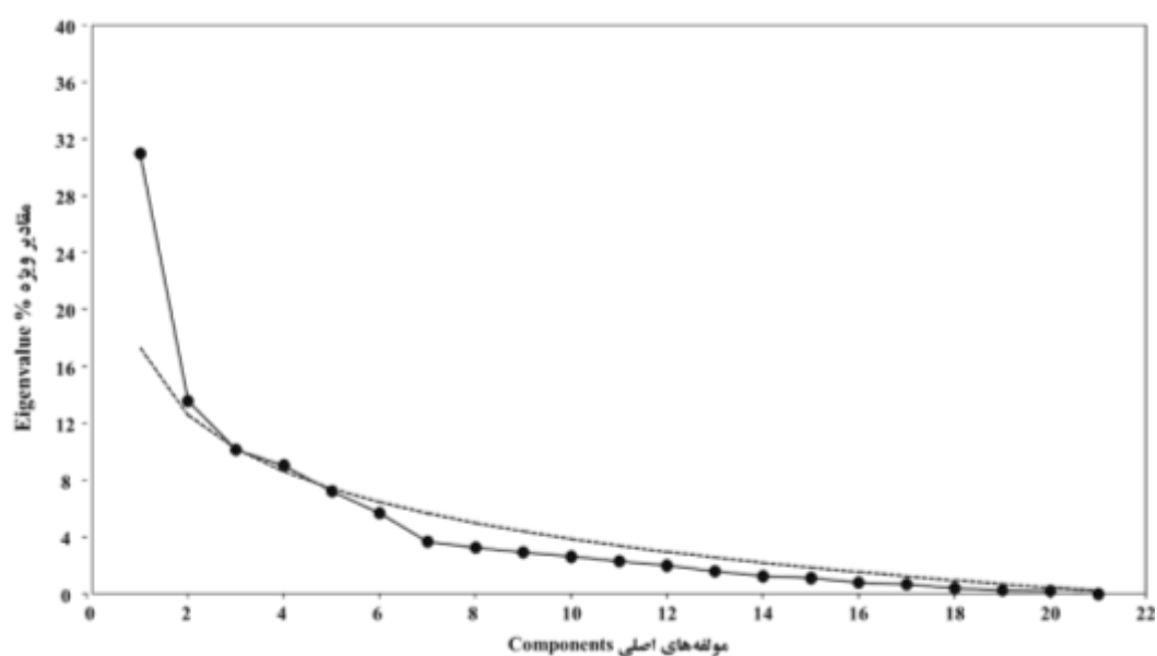
شکل ۳. نمودار سنگریزه‌ای مؤلفه‌های اصلی صفات اندازه‌زی و خط‌چین، جداکننده مؤلفه‌های اصلی معنی‌دار بر اساس حد برش جولیف
