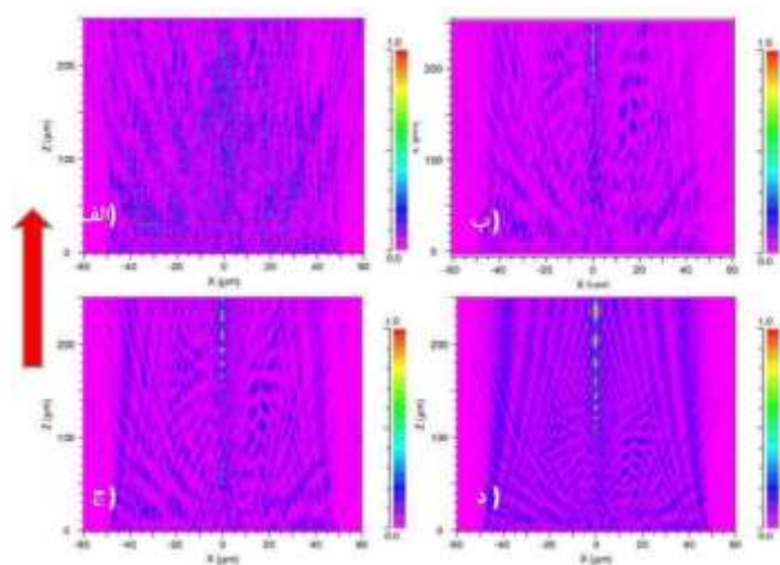
شکل ۵. توزیع فضایی توان عبوری برای طول موج‌های (الف) \lambda = 280 \text{ nm} ، (ب) \lambda = 532 \text{ nm} ، (ج) \lambda = 633 \text{ nm} ، (د) \lambda = 1 \text{ }\mu\text{m} در پیچه از z = -0.6 \text{ }\mu\text{m} تا z = 0.4 \text{ }\mu\text{m} کشیده شده است. فلش قرمز رنگ در جهت انتشار نور ورودی است و توان مربوط به زمینه ورودی (a.u.) 0.08 در نظر گرفته شده است (De Tommasi et al., 2010).
