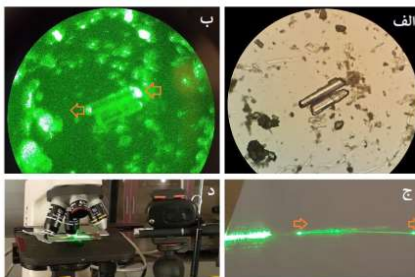
شکل ۱۰. (الف) دو دیاتوم استوانه‌ای (ب) تابش لیزر سبز به دیاتوم‌های استوانه‌ای (ج) تابش لیزر سبز به تار نوری (د) چینه‌ش آزمایش تابش لیزر به اسلاید حاوی دیاتوم. پیکان‌های قرمز جهت ورود و خروج نور به موج‌بر را نشان می‌دهد.
