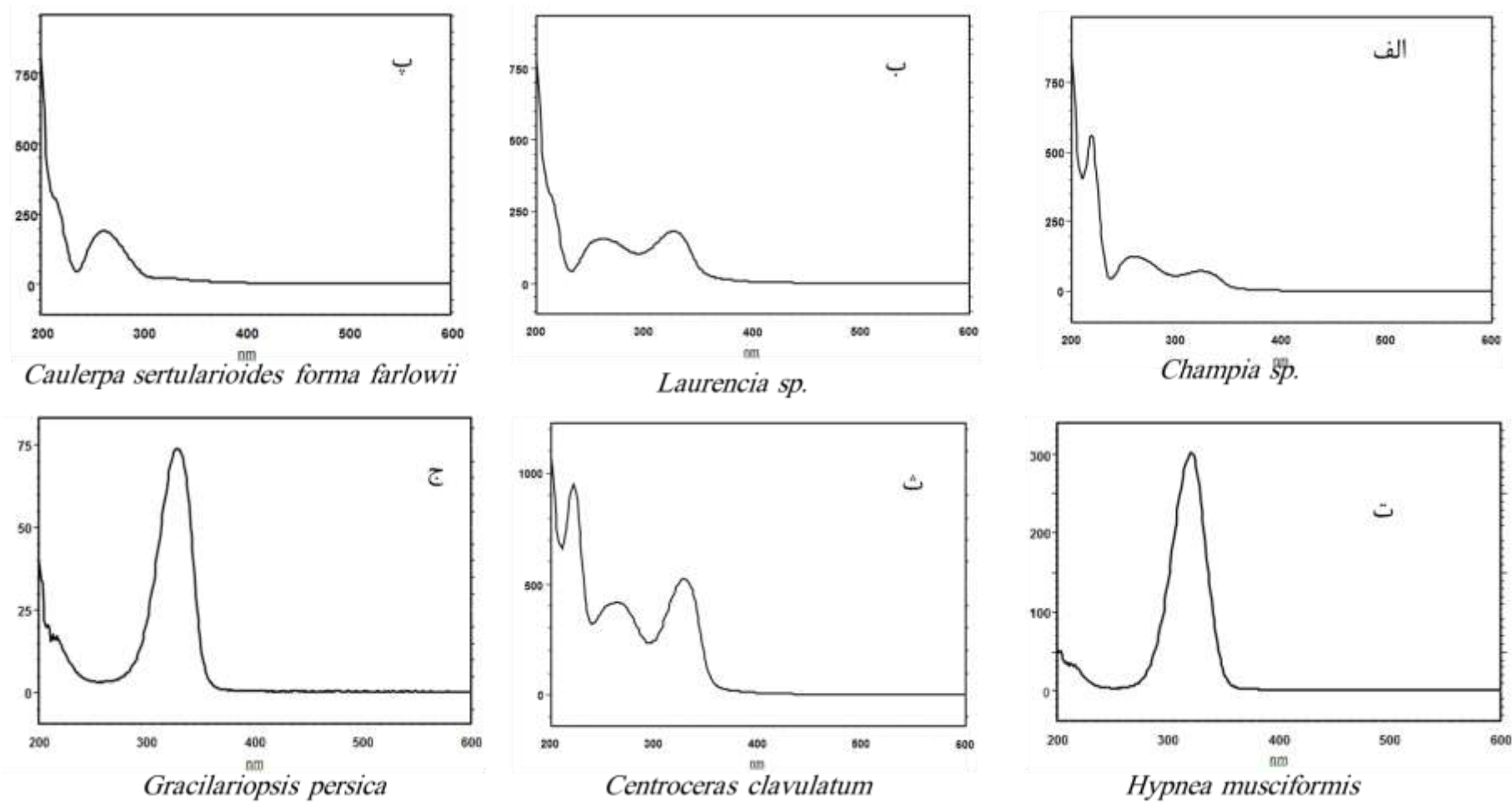
شکل ۳. طیف ماوراءبنفش (UV) عصاره نیمه خالص MAAs استخراج شده از ماکرو جلبک‌های خلیج فارس
