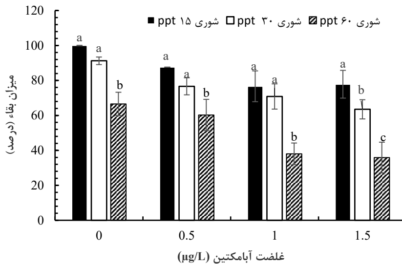
شکل ۶. بقاء ناپلیوس‌های A. franciscana پس از ۲۴ ساعت تماس با آبامکتین و سپس قرارگیری در محیط‌های با شوری مختلف در دوره‌ی بازیابی. *حروف روی ستون‌ها نشان‌دهنده تفاوت معنی‌دار بین تیمارها در همان غلظت می‌باشند.
