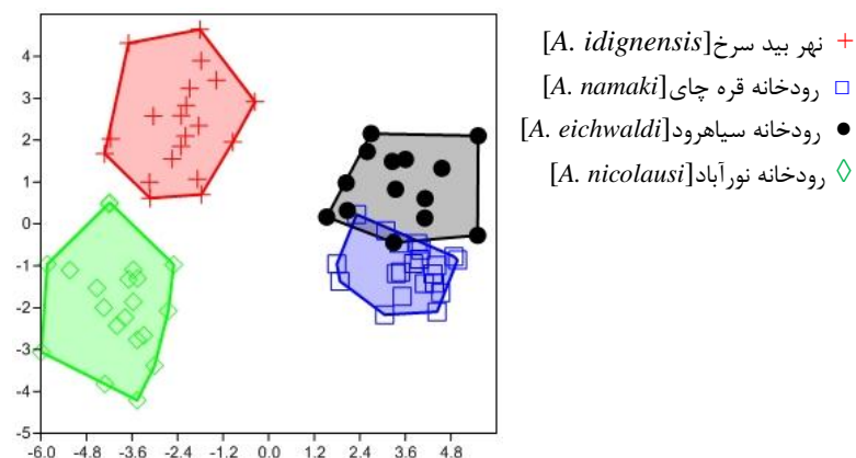
شکل ۶. نمودار پراکنش افراد براساس آزمون CVA صفات ریخت سنجی نسبی گونه‌های مورد مطالعه
