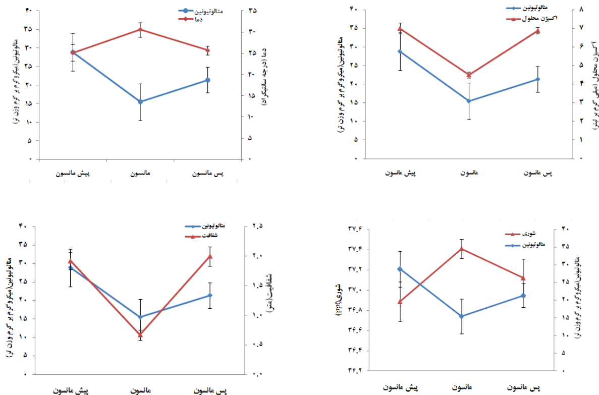
شکل ۳. مقایسه تغییرات میانگین دما، اکسیژن محلول، شوری و شفافیت نسبت به سطوح ماتالوتیونین در طی سه فصل پیش مانسون، مانسون و پس مانسون
