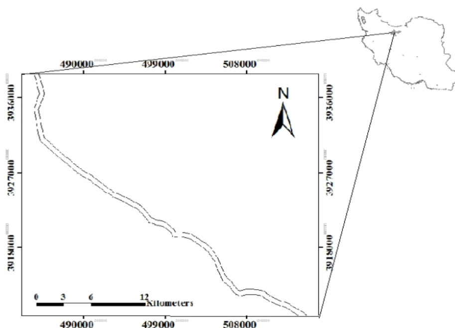
شکل ۱. موقعیت جغرافیایی منطقه نمونه برداری (رودخانه شور کرج، استان البرز)
