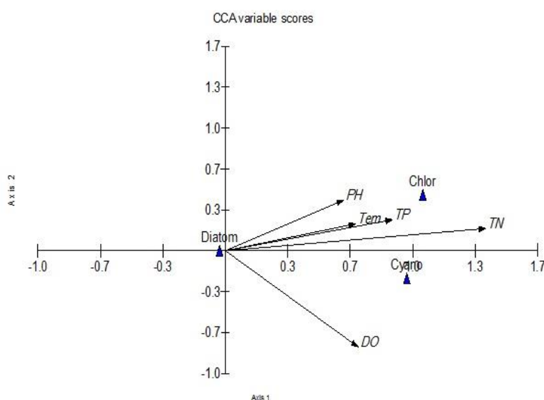
شکل ۶. اولین و دومین محور CCA برای فراوانی فیتوپلانکتون و عوامل محیطی در رودخانه کن، سال ۱۳۹۳
