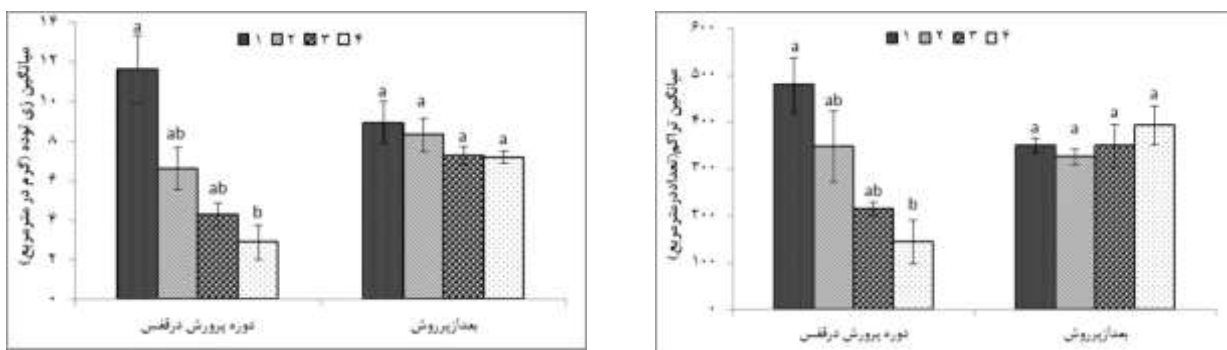
شکل ۴. میانگین تراکم (تعداد در مترمربع) و زی‌توده (گرم در مترمربع) ماکروبن‌توزهای سد گلستان یک در ایستگاه‌های مختلف در طی پرورش ماهی در قفس و بعد از پرورش در سال ۹۶-۱۳۹۵.
