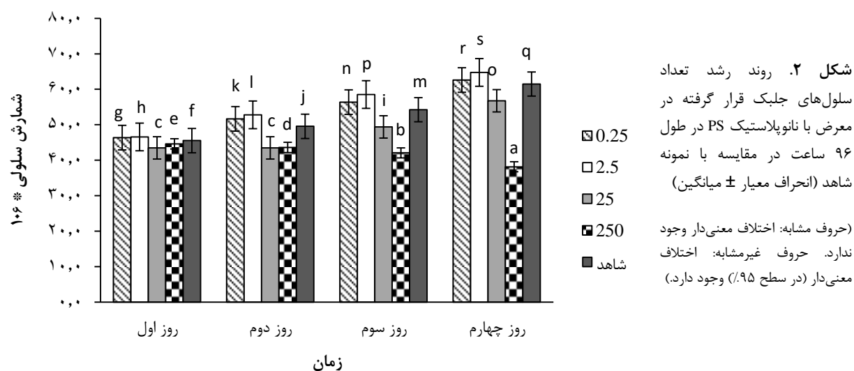
شکل ۲. روند رشد تعداد سلول‌های جلبک قرار گرفته در معرض نانوپلاستیک PS در طول ۹۶ ساعت در مقایسه با نمونه شاهد (انحراف معیار \pm میانگین)
