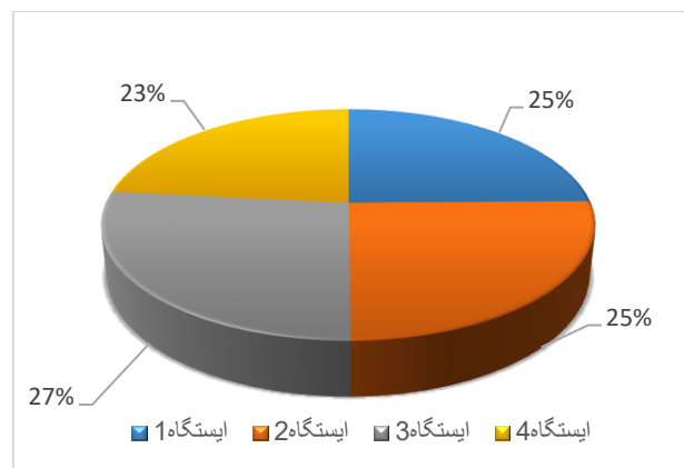
شکل ۱. میانگین درصد فراوانی جوامع فیتوپلانکتونی در ایستگاه‌های مورد مطالعه دریاچه کارون ۴ در طول مراحل نمونه‌برداری
